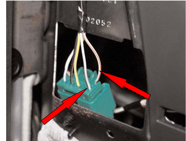
Grüner Stecker hinter der linken Seitenabdeckung des Armaturenbretts. CAN hi - Pin 9 (weiß/grau) CAN lo - Pin 1 (weiß/orange)
