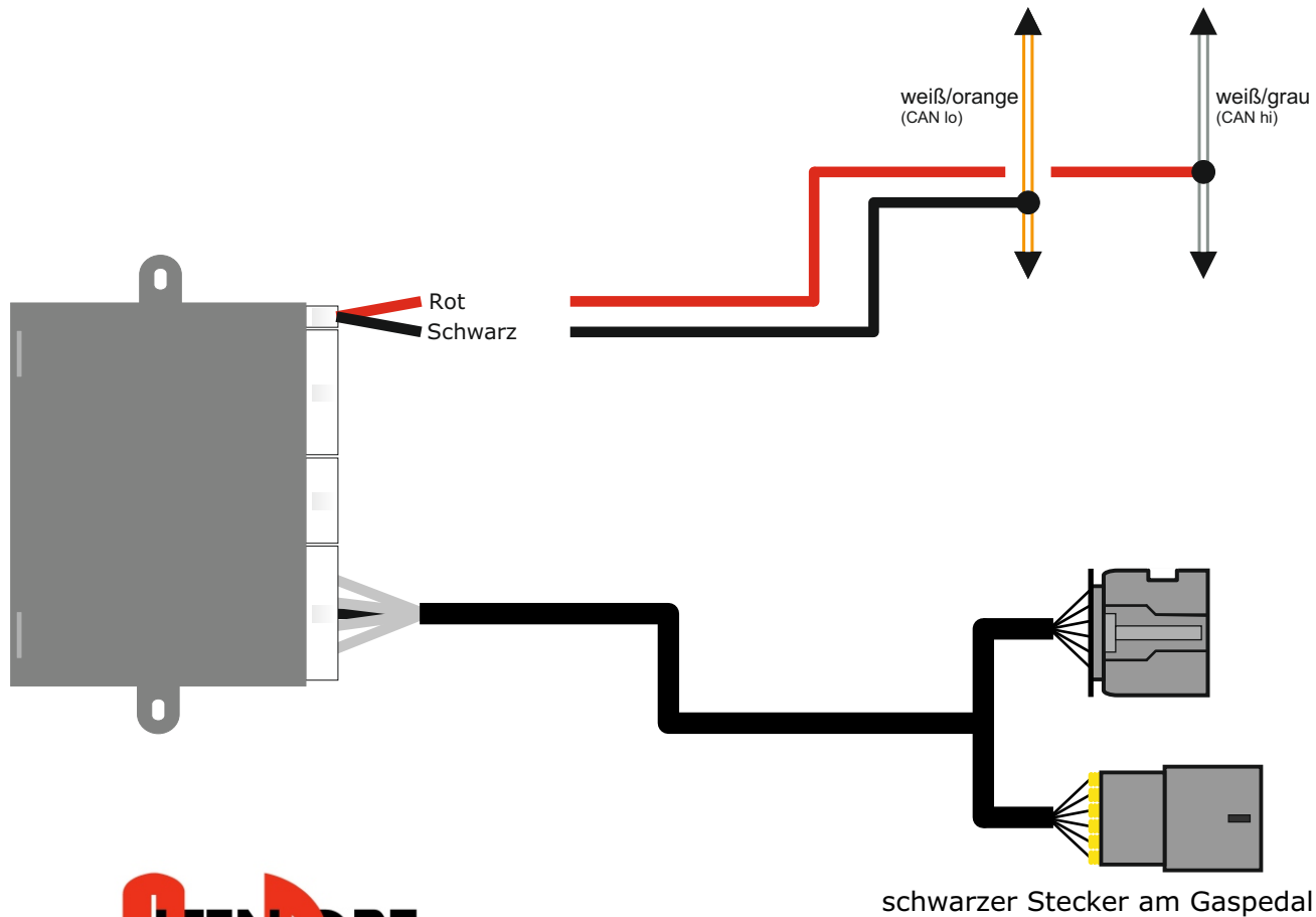
Grüner Stecker hinter der linken Seitenabdeckung des Armaturenbretts. CAN hi - Pin 9 (weiß/grau) CAN lo - Pin 1 (weiß/orange)
